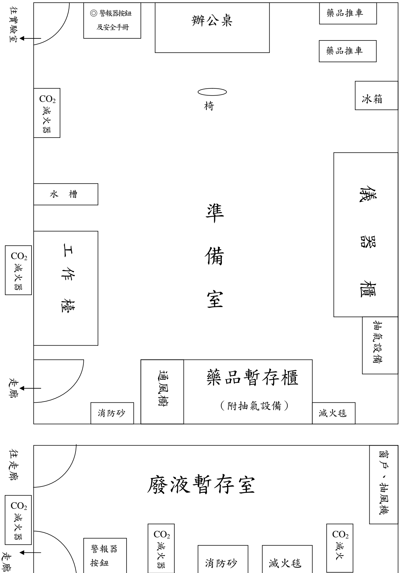
參考 99 課程綱要設備標準之準備室與廢液暫存室參考圖
