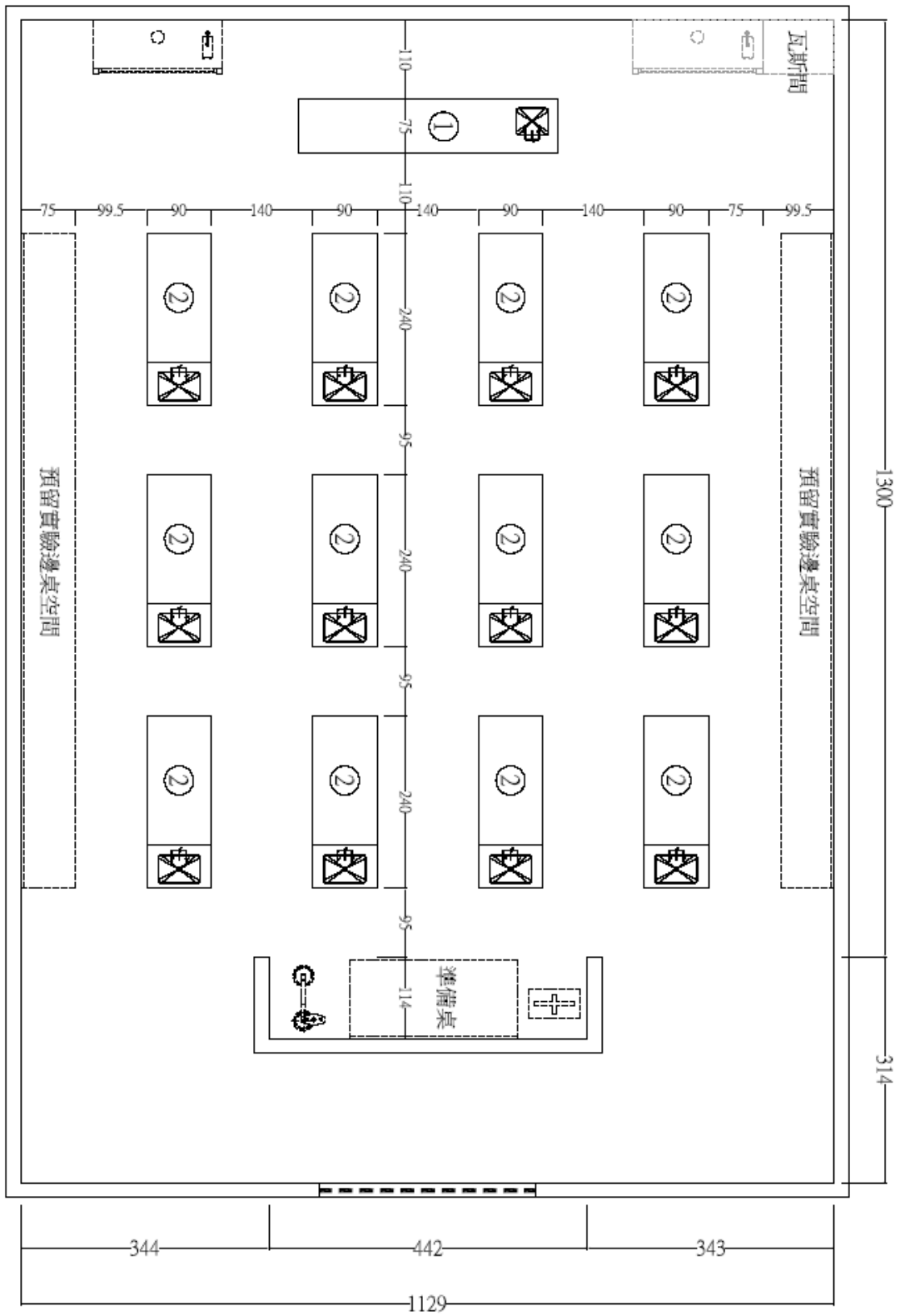
①實驗室設備配置平面圖
